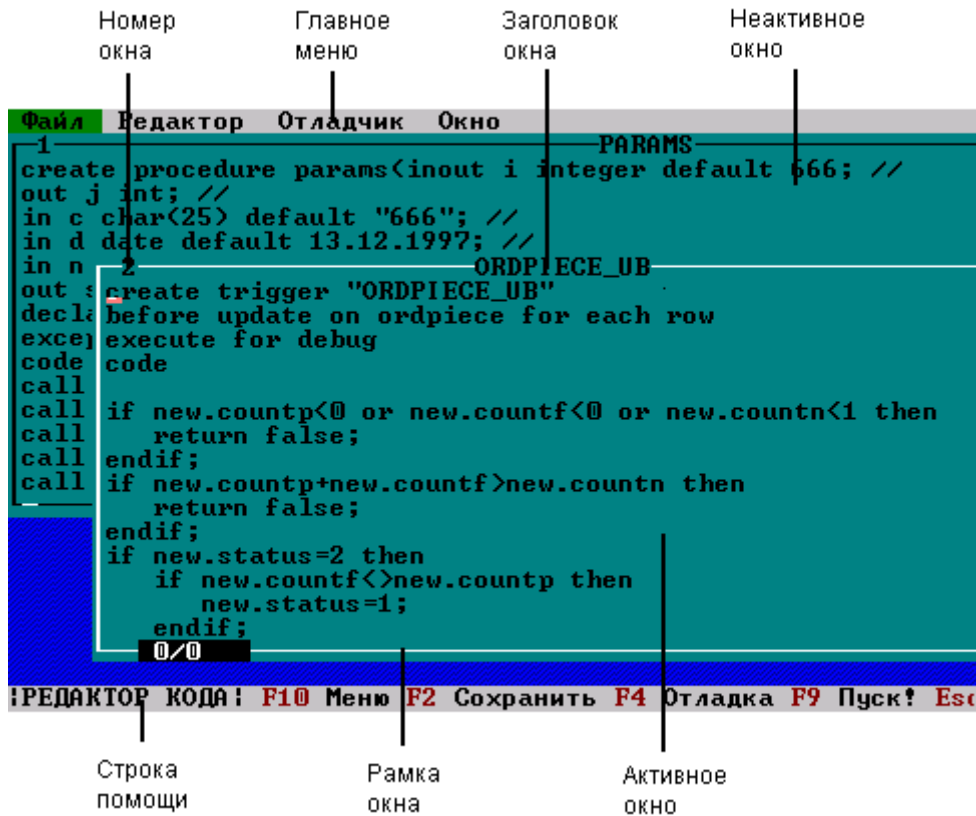
Рис. 3. Отладчик с двумя открытыми объектами отладки
