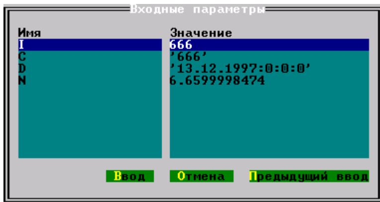
Рис. 8. Окно ввода параметров процедуры
